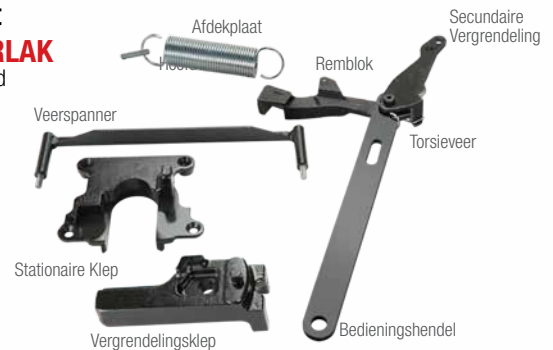
Vergrendelingsklep
